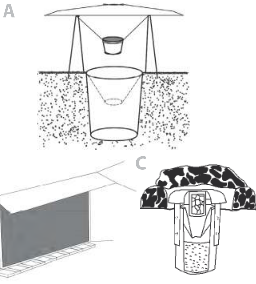
Figura 14: A. modelo de trampa Pitfall no letal, B. trampa de interceptación aérea (TIA) y C. necrotrampa NTP 80 (redibujado de Morón & Terrón 1984).
